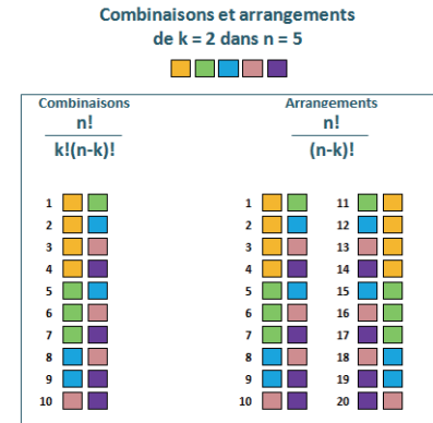
Figure 14–40 Choix de deux éléments parmi cinq (symbolisés par les carrés de couleur). Si l'on tient compte de l'ordre dans lequel on a choisi les deux éléments, on a 20 choix possibles, si l'on n'en tient pas compte, le nombre de possibilités est réduit à 10.
