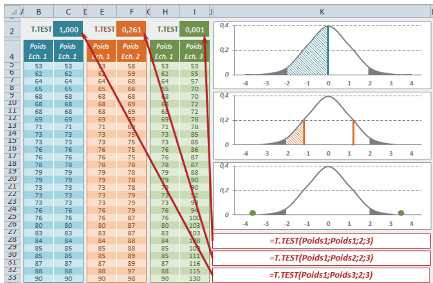
Figure 15-84 Poids des 29 individus de trois échantillons tirés de villes différentes
