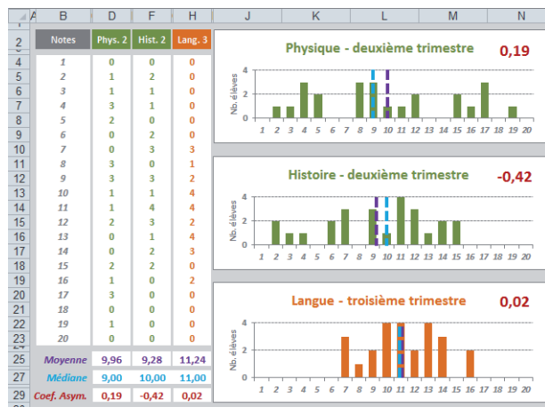
Figure 15-14 La formule qui permet de calculer le coefficient d'asymétrie d'une distribution utilise sa moyenne et son écart-type ( \sigma ).
