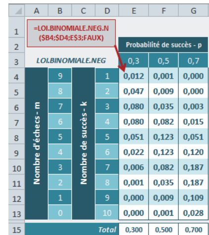
Figure 15-36 Mise en œuvre de la fonction LOI.BINOMIALE.NEG.N. Cette fonction applique la formule indiquée figure 15-37.
