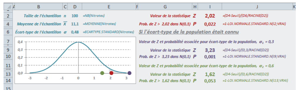
Figure 15-89 À partir de la définition du test, calcul de la statistique Z pour l'échantillon étudié
